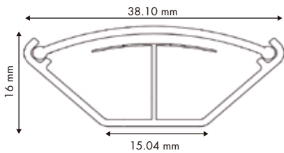
CANAL 90° CON DIVISIÓN
